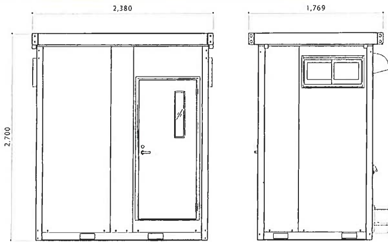
立面図
